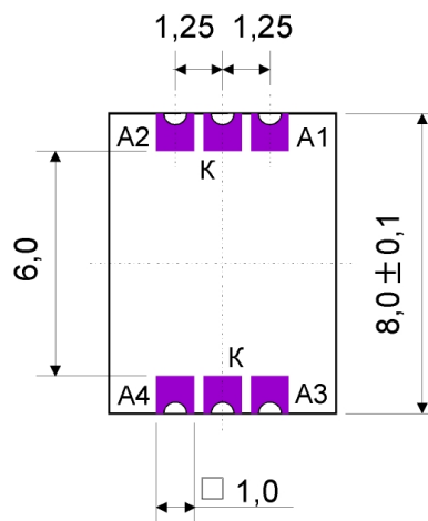
Четырехэлементная фотодиодная сборка СФД4-02
