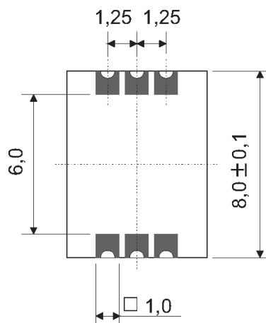
Четырехэлементная фотодиодная сборка СФД4-01
